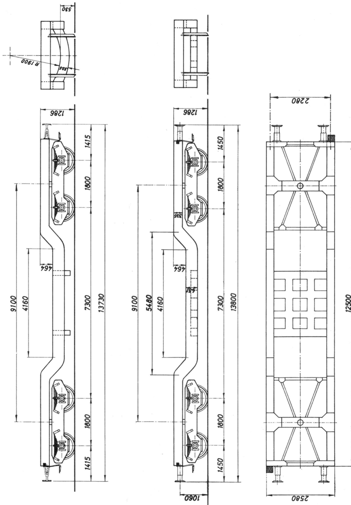
Tegninger fra DSB DRM II. Øverst (til venstre) udseende før 1936. Nederst (til højre) med ny vognbund fra 1936 og cylinderpuffere fra 1966. Håndbremsen på højre bogie samt mange andre detaljer er udeladt. Tilnærmet skala 1:87.
